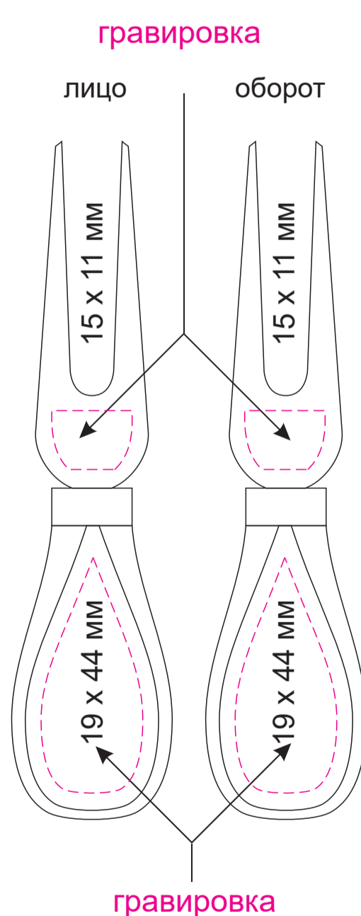
Нож-вилка
