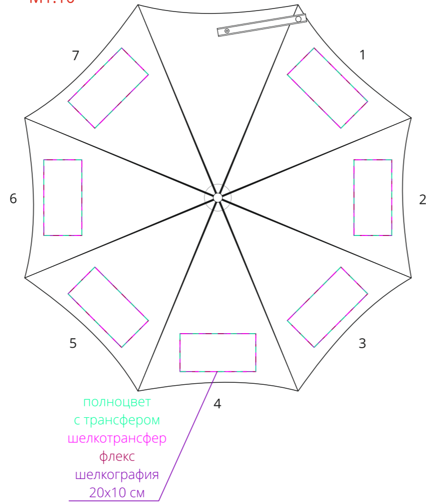
купол M1:10
