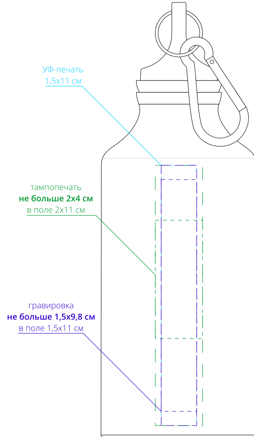
сторона b
