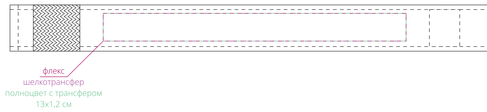
хлястик M1:1
